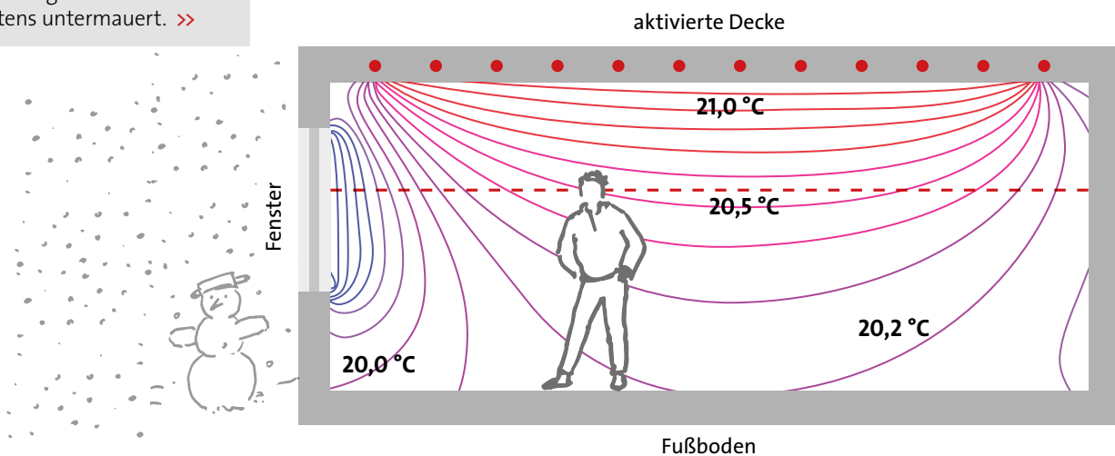
Abb. 5 | Vertikalschnitt durch einen Musterraum mit Isothermen im Heizfall/Winterbetrieb bei aktivierter Decke. Auffällig sind die gleichmäßige Temperaturverteilung und die geringen Temperaturunterschiede im Raum. © Z + B
