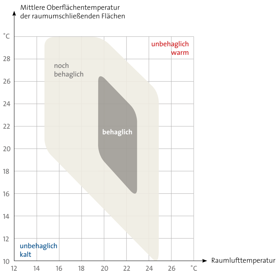
Abb. 6 | Behaglichkeitsbereich Oberflächentemperatur zu Lufttemperatur. © z + b
