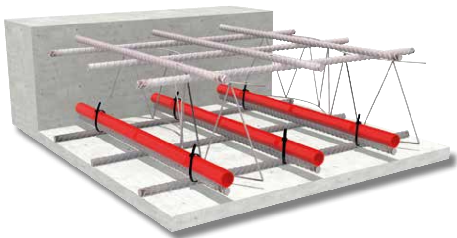
Abb. 2 | Schemaskizze Bauteilaktivierung einer Geschoßdecke. © Z + B
